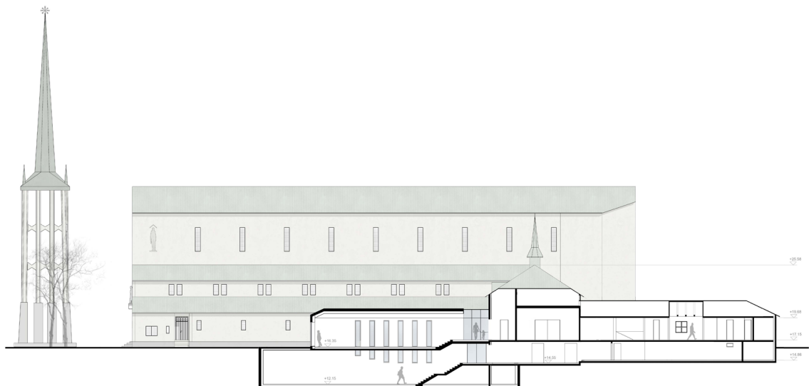
Snitt A-A
